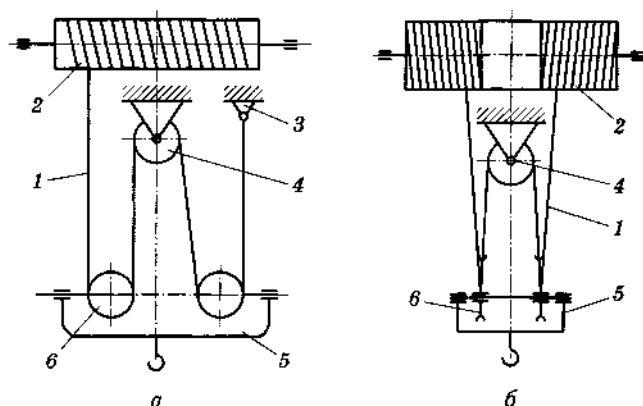
Рис. 2.6. Канатные полиспасты:
