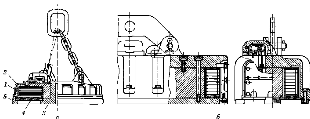
Рис. 2.10. Грузоподъемные электромагниты:
