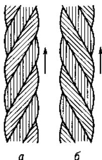
Рис. 2.2. Направление свивки:
