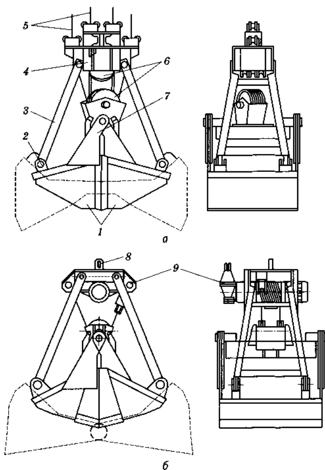
Рис. 2.9. Грейфер:
