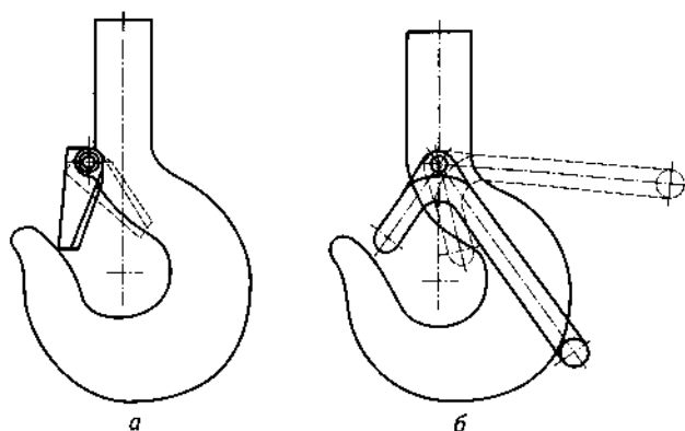
Рис. 2.8. Замки предохранительные для однорогих крюков:
