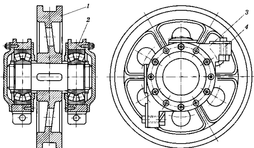
Рис. 2.11. Двухреборное ходовое колесо на угловой буксе:
