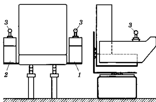
Рис. 4.4. Кресло-пульт «РАДУК»:
