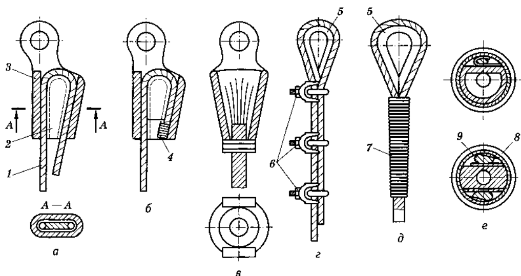
Рис. 2.4. Крепление концов канатов в конусной втулке клином (а, б), заливкой легкоплавким сплавом (в), с помощью зажимов (г), заплеткой (д), на барабане (е):
