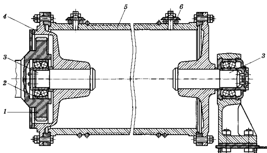
Рис. 2.5. Барабан грузовой лебедки:
