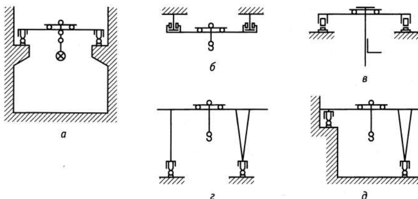
Рис. 1.1. Конструкции кранов мостового типа:
