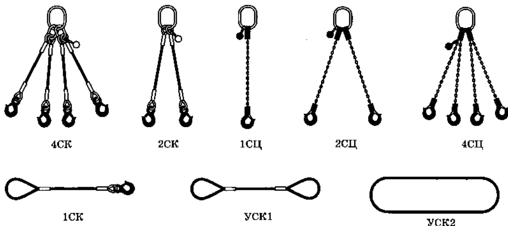
Рис. 5.1. Стропы для подъема и перемещения грузов (цифры перед буквенными обозначениями стропов означают число ветвей):
