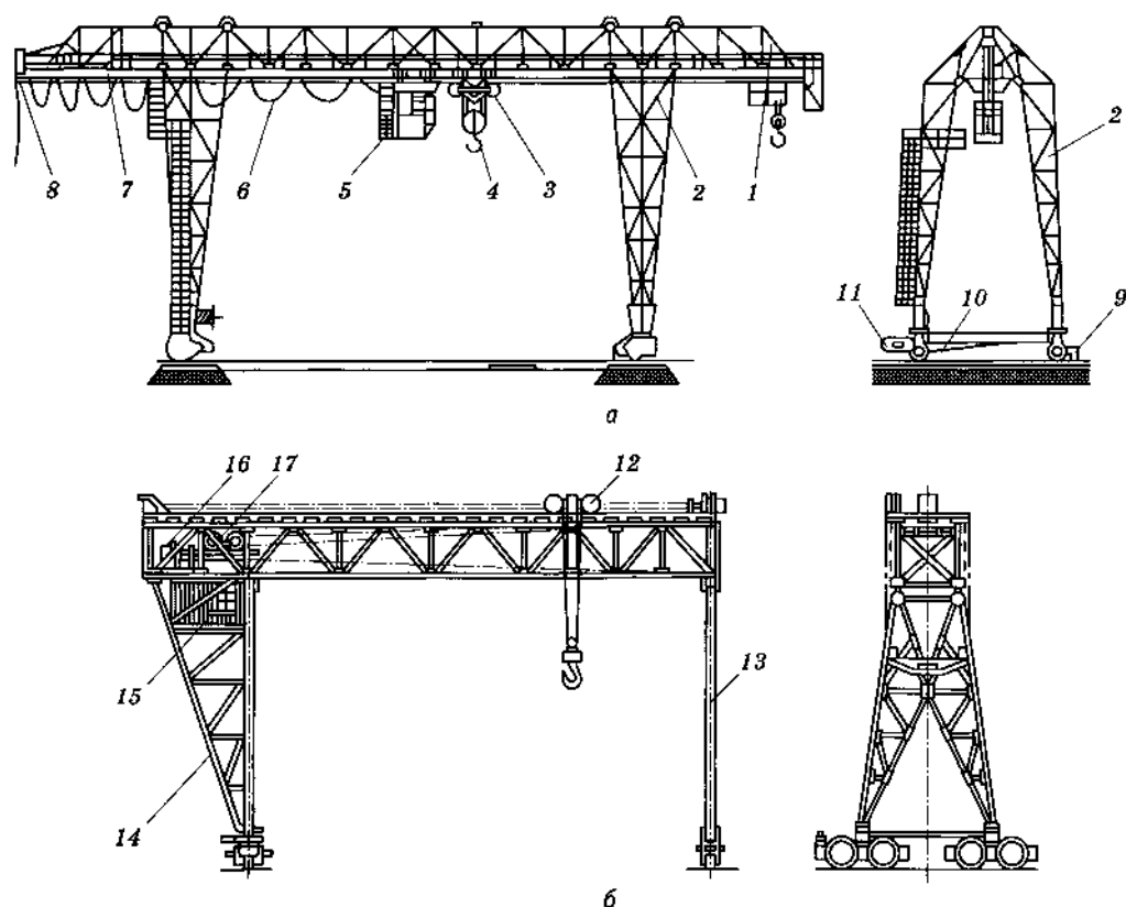
Рис. 1.4. Козловые краны:
