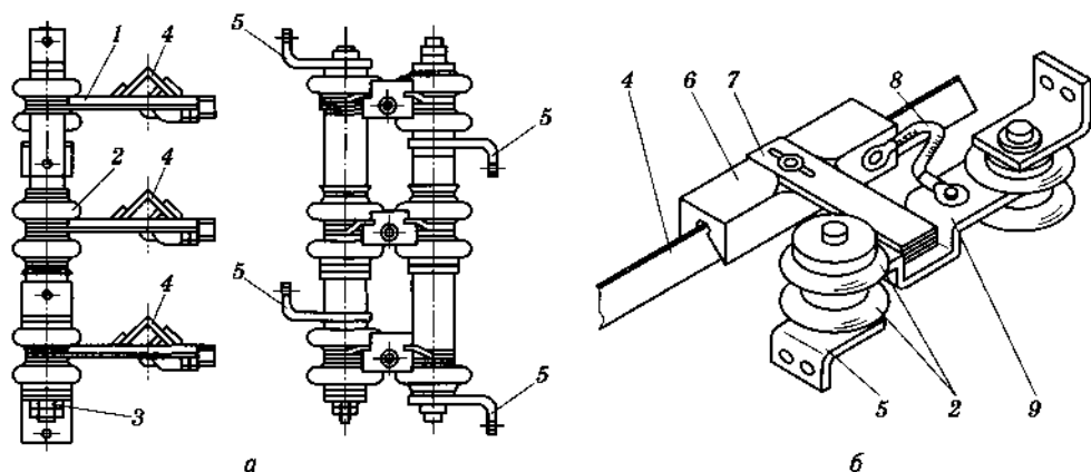
Рис. 4.1. Троллейный токоподвод:
