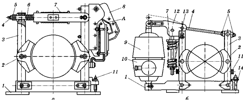
Рис. 2.12. Тормоз колодочный ТКТ с электромагнитом марки МО (а) и ТКТ с электрогидравлическим толкателем (б):
