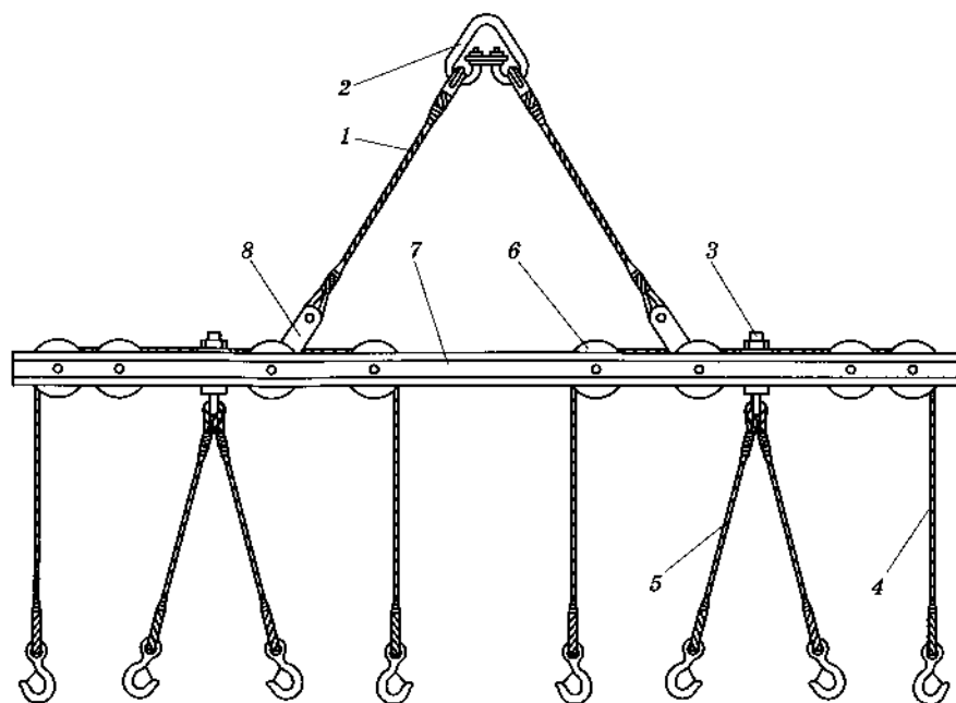
Рис. 5.2. Балансирная траверса:
