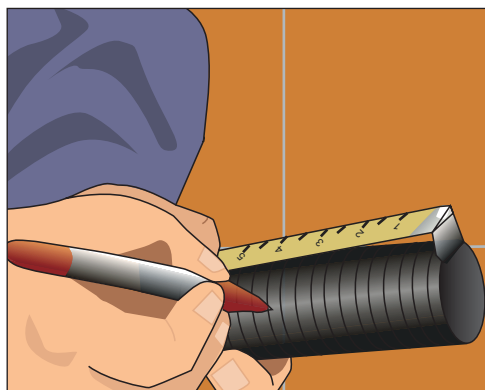
Рис. 10.130. Отмеряем нужную длину отводной трубы сифона
