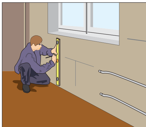
Рис. 12.56. Делаем отметки крепления радиатора
