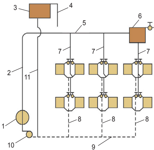
Рис. 12.40. Схема водяного отопления с принудительной циркуляцией ( нижняя разводка ):
