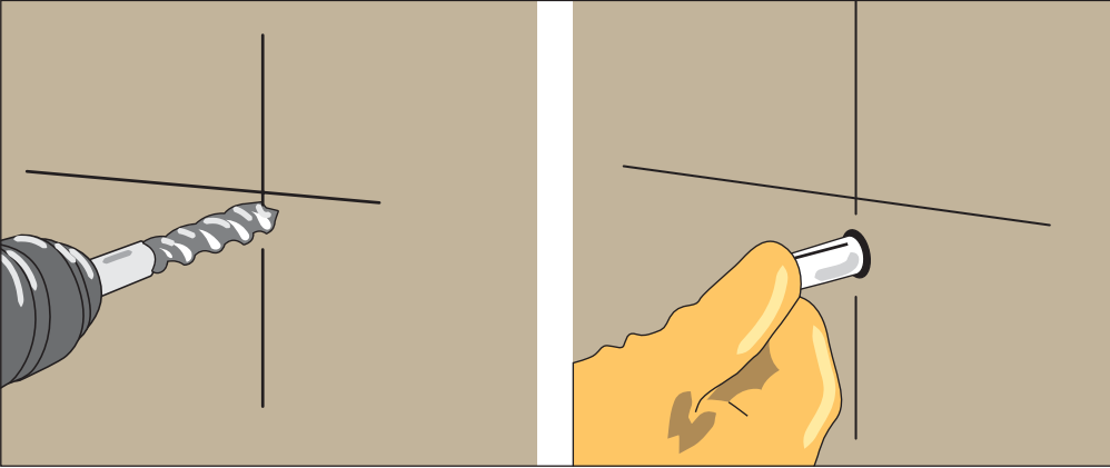
Рис. 12.58. Просверливаем отверстия (слева), вставляем дюбели (справа)
