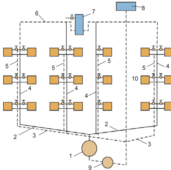
Рис. 12.39. Схема водяного отопления с принудительной циркуляцией ( верхняя разводка ):
