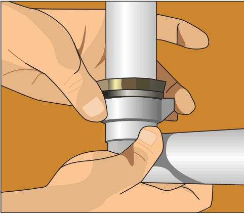
Рис. 11.52. Отсоединяем сифон
