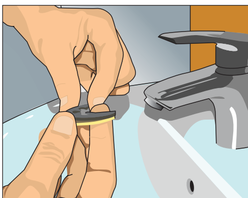
Рис. 10.29. Подкладываем под прижимную пластину резиновую прокладку; вставляем на шпильки и закручиваем гайки на шпильках, зажимаем их крепко ключом
