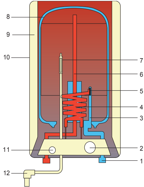
Рис. 10.280. Устройство накопительного водонагревателя: 1 — труба для забора холодной воды; 2 — регулятор температуры; 3 — теплообменник; 4 — нагревательный элемент (ТЭН); 5 — предохранительный элемент; 6 — труба вывода горячей воды; 7 — температурный датчик; 8 — внутренняя емкость; 9 — теплоизолирующий наполнитель; 10 — корпус; 11 — контрольный датчик (лампочка); 12 — кабель
