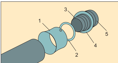
Рис. 4.73. Пресс-фитинг: 1 — обжимная гильза; 2 — пластиковое диэлектрическое кольцо; 3 — уплотнительные кольца; 4 — фиксатор гильзы; 5 — корпус
