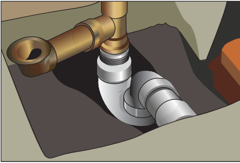
Рис. 10.177. Тройник
