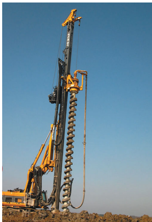
Рис. 4.3. Бурение артезианской скважины
