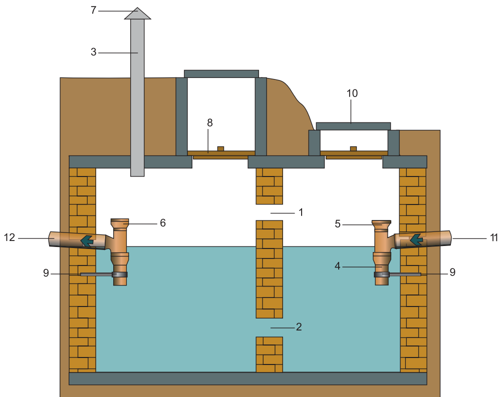
Рис. 8.30. Устройство кирпичного септика: 1 — воздушное отверстие 250 \times 250 мм; 2 — переливное отверстие 250 \times 250 мм; 3 — вентиляционная труба; 4 — удлиняющий чугунный патрубок; 5 — впускной тройник; 6 — выпускной тройник; 7 — флюгарка; 8 — утепленная деревянная крышка; 9 — крепежный хомут; 10 — крышка люка; 11 — подводящий трубопровод диаметром 100 мм; 12 — отводящий трубопровод диаметром 100 мм
