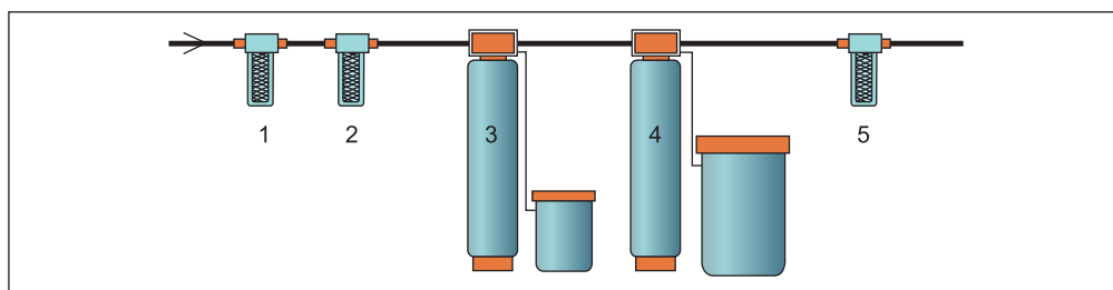
Рис. 7.2. Использование фильтров: 1 — фильтр механической очистки; 2 — фильтр тонкой очистки; 3 — установка обезжелезивания; 4 — установка умягчения; 5 — угольный фильтр
