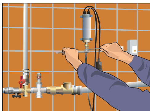
Рис. 4.27. Подсоединяем подводку к прибору с помощью гаечных ключей
