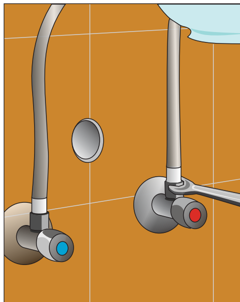
Рис. 10.48. Гибкие шланги прикручиваем к угловым вентилям с помощью гаечного ключа
