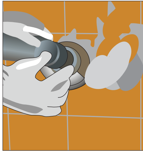
Рис. 10.37. Убираем старые шурупы с резьбой угловой шлифовальной машинкой с отрезным диском по металлу
