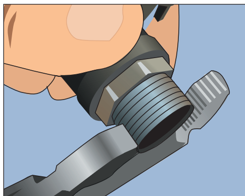
Рис. 1.19. Подготавливаем трубу к наматыванию льна (при необходимости наносим резьбу)
