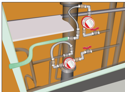
Рис. 6.9. Установленные счетчики готовы к опломбированию
