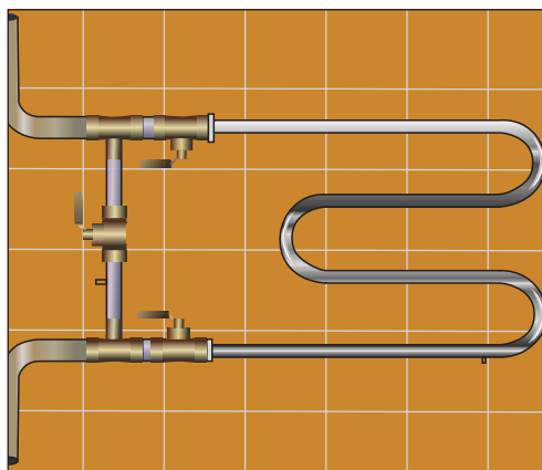
Рис. 12.72. Установленный байпас
