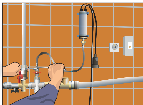
Рис. 4.28. Подсоединяем второй конец шланга к крану водоснабжения
