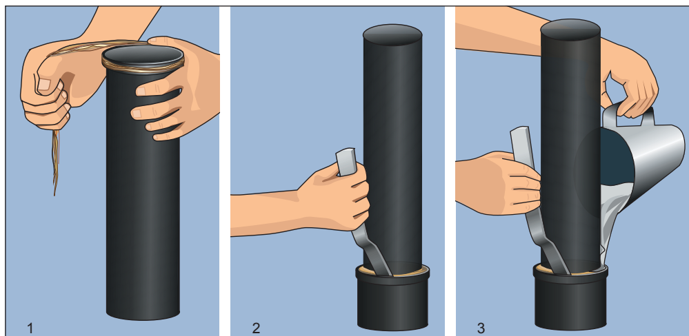
Рис. 1.47. Заделка стыков чугунных канализационных труб: 1 — намотка льняных прядей; 2 — осадка прядей; 3 — заделка асбестоцементным раствором
