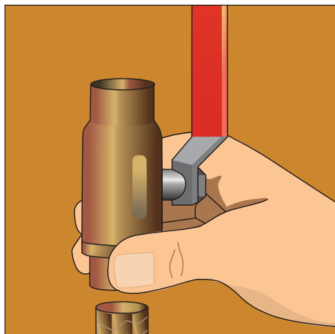
Рис. 10.292. Устанавливаем запорный вентиль на «входе» для холодной воды и на «выходе» — для горячей
