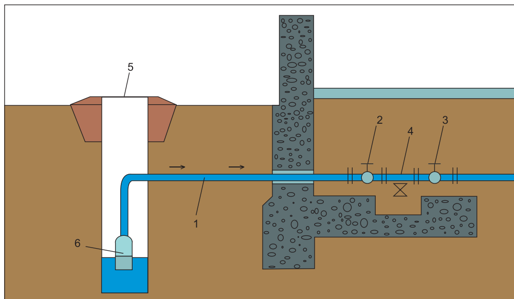
Рис. 5.3. Схема прокладки водопровода сквозь фундамент: 1 — ввод, диаметр трубы не менее 50 мм; 2 — первый вентиль; 3 — второй вентиль; 4 — спускной кран; 5 — колодец; 6 — насос
