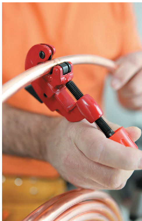
Рис. 4.47. Резка медных труб роликовым труборезом
