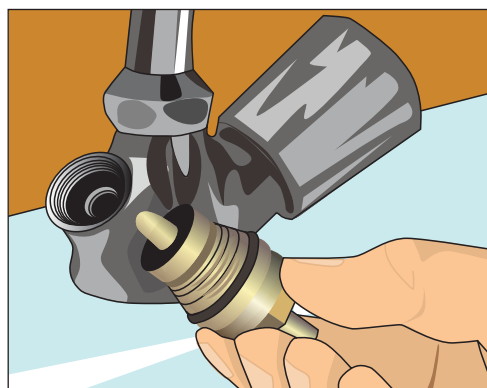
Рис. 11.34. Прочищаем все внутри, удаляем накопившиеся отложения
