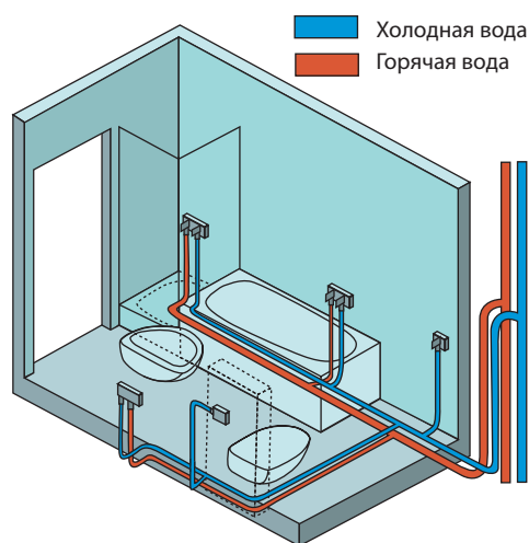
Рис. 4.10. Тройниковая схема разводки водопровода
