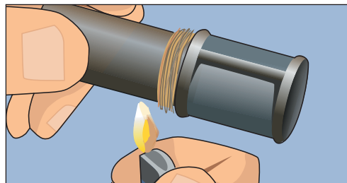
Рис. 1.28. Удаляем лишние волокна льна с помощью огня
