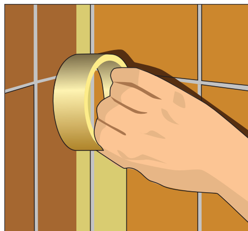
Рис. 1.42. Оклеиваем поверхность стыка самоклеящейся лентой
