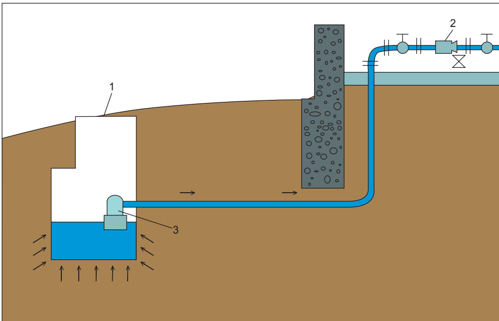
Рис. 5.2. Схема прокладки водопровода под фундаментом: 1 — каптажная камера; 2 — водомет; 3 — насос
