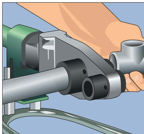
Рис. 4.61. Вставляем элементы пластикового водопровода в сварочный аппарат
