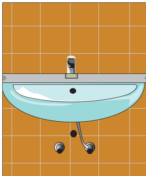
Рис. 10.47. Выравниваем раковину с помощью уровня
