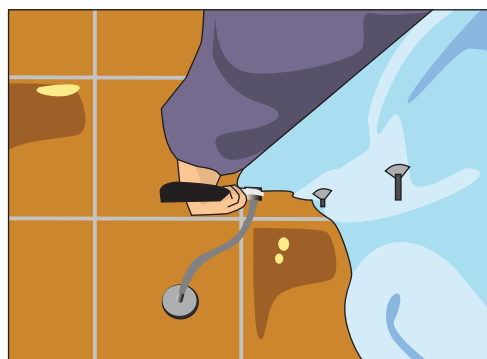
Рис. 10.83. Отсоединяем подводящий шланг (откручиваем гайку рожковым ключом 19 × 22)
