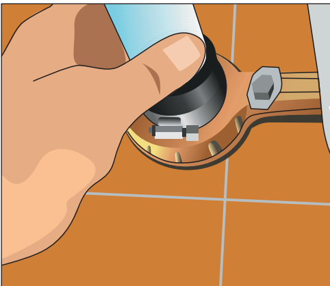
Рис. 10.134. Соединяем цельнолитый сифон с раструбом канализации
