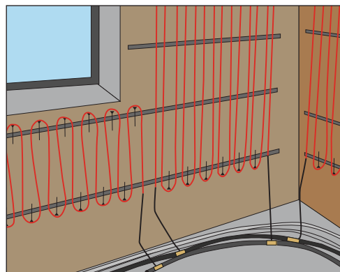
Рис. 12.17. Укладка теплых стен по периметру комнаты
