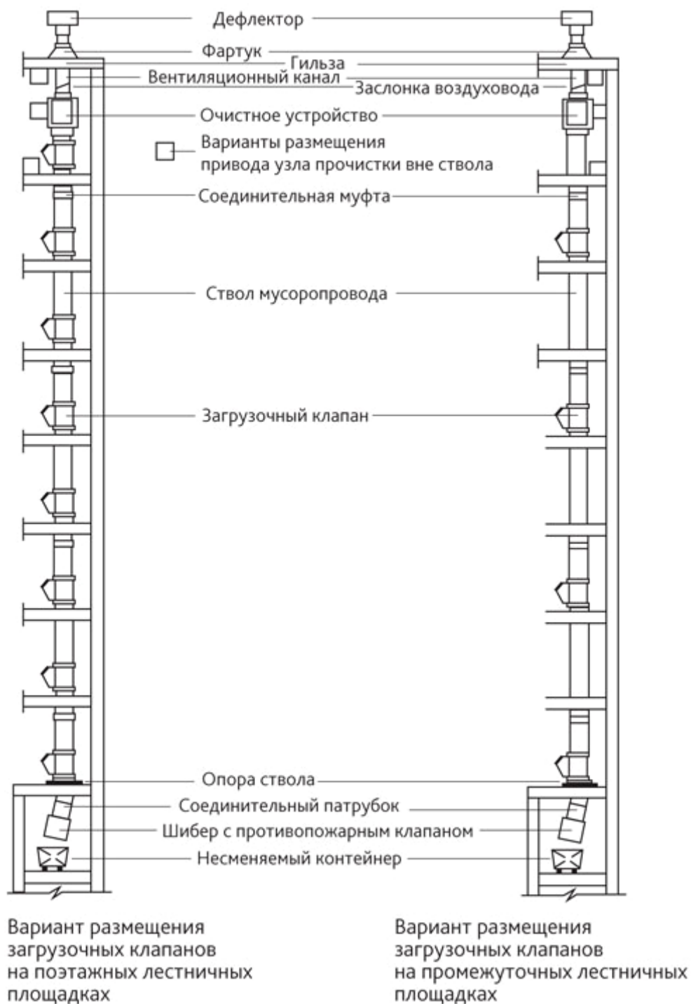
Устройство мусоропровода
