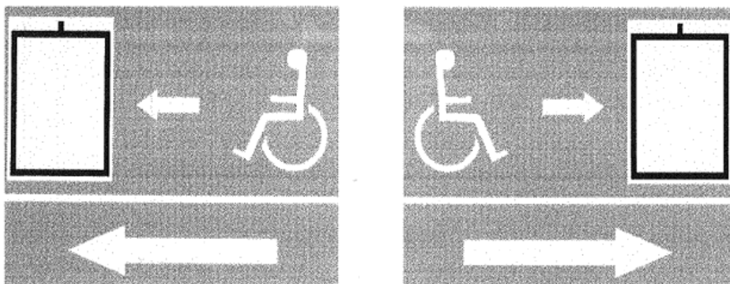
Пиктограмма для эвакуационного лифта
