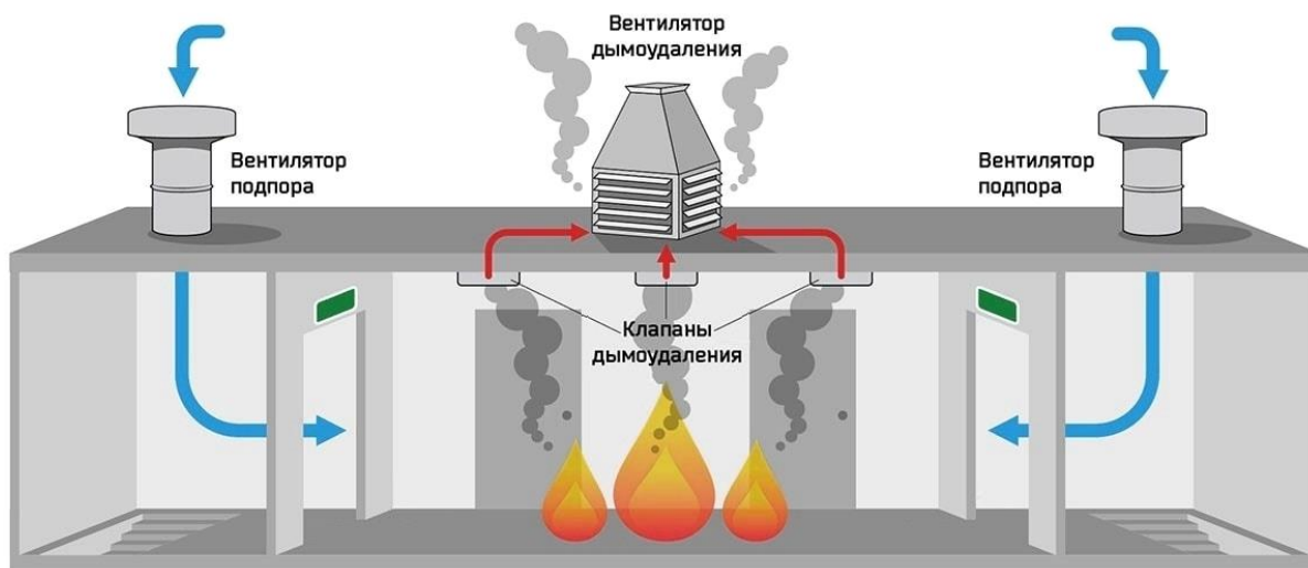
Схема дымоудаления
